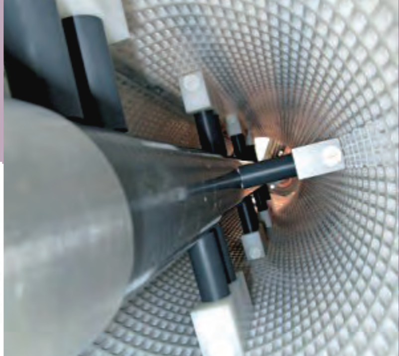
Incollaggio filtri - Gluing filters
